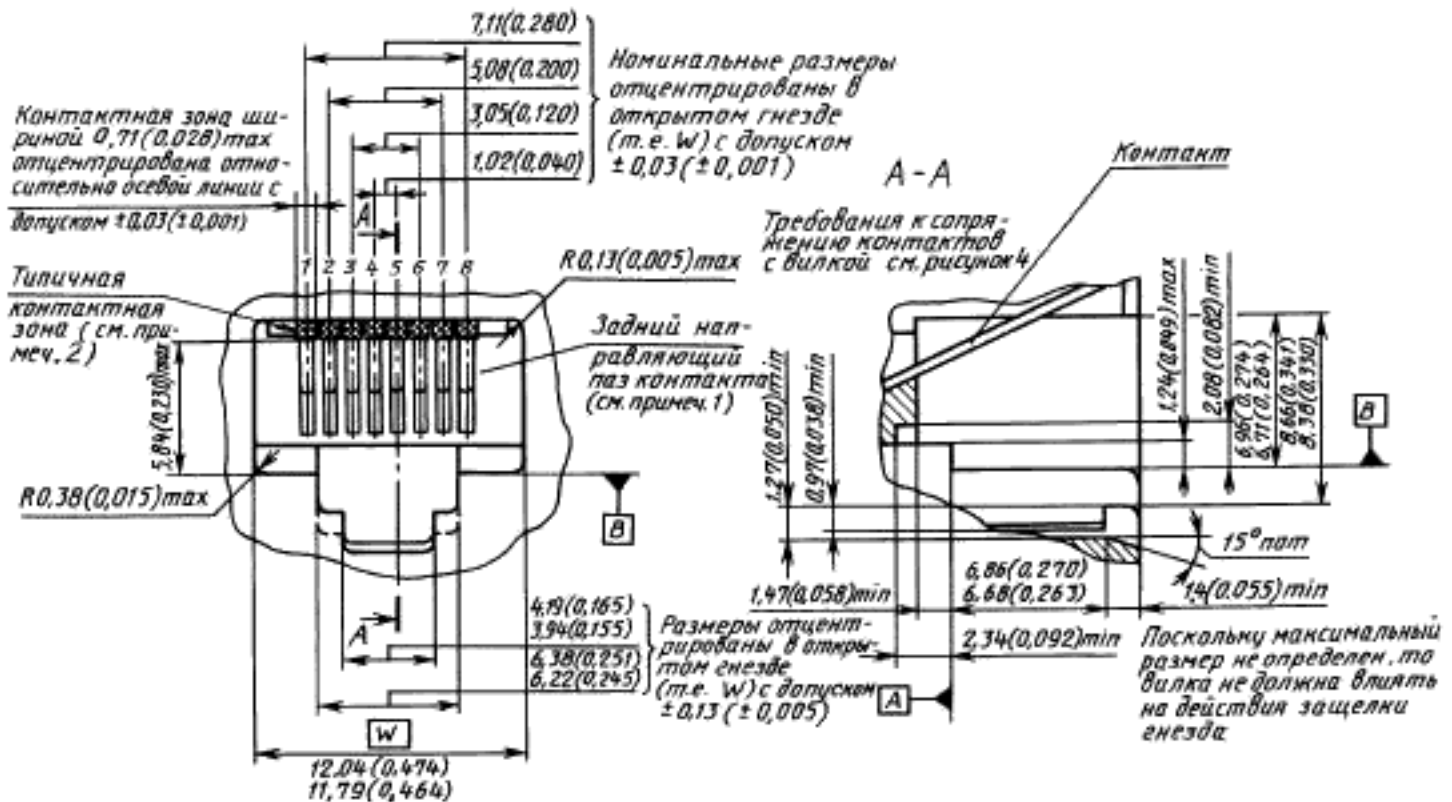
Рисунок 5 — Механические характеристики гнезда
