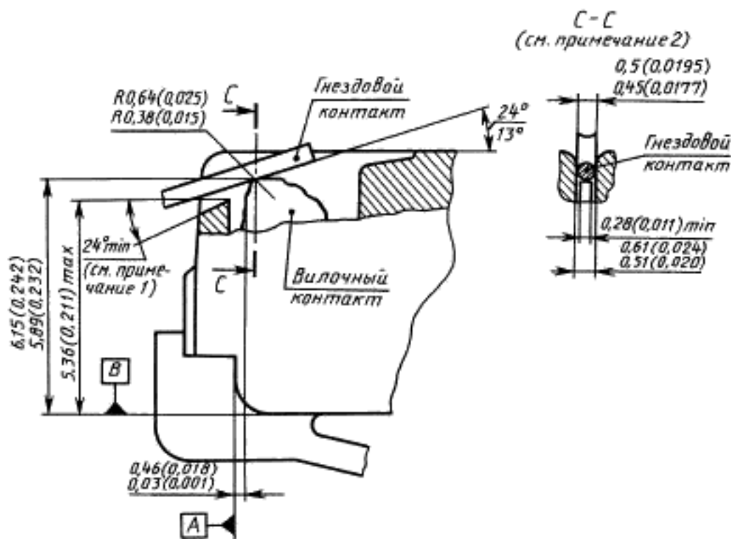
Рисунок 4 — Спецификация контактов гнезда и вилки
