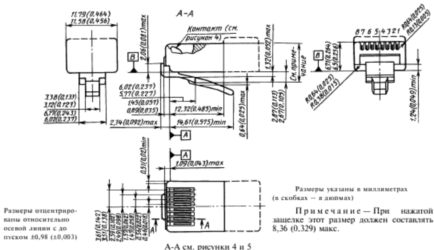
Рисунок 3 — Механические характеристики вилки
